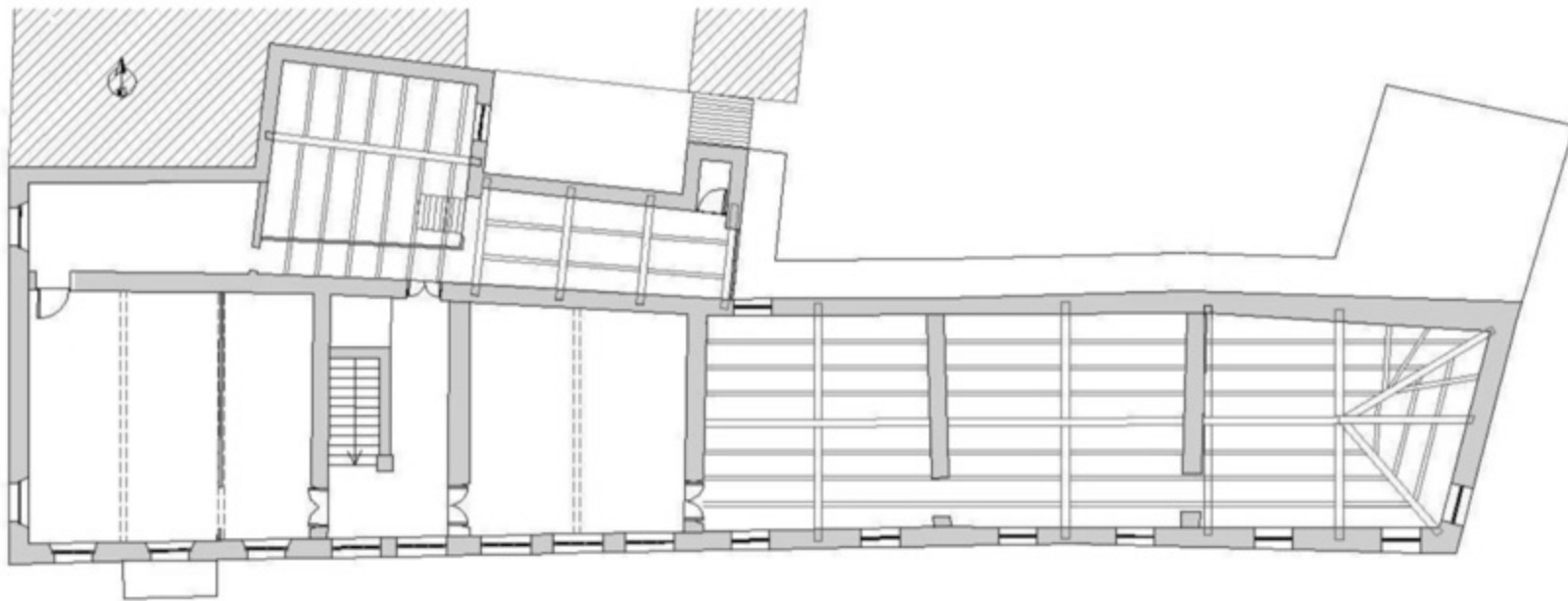
Fig. 94 - Pianta del piano secondo
