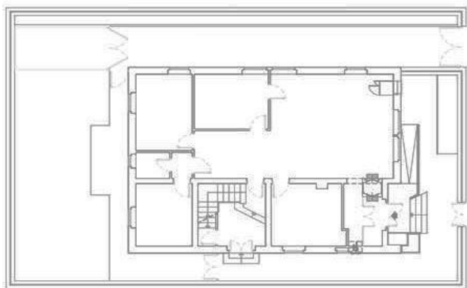
Pianta PT
